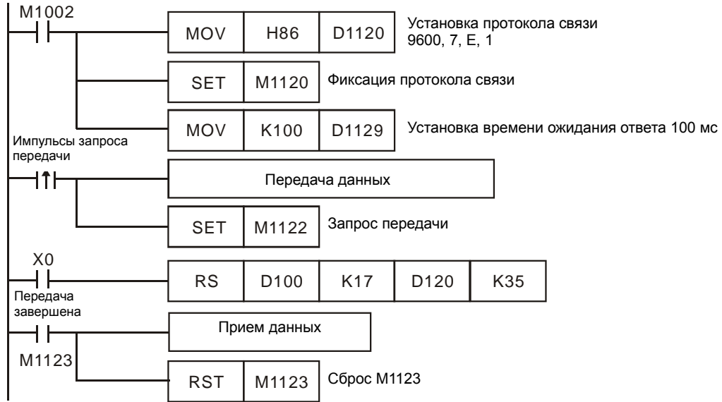
Регистры для передачи данных (ПЛК передает сообщение)
