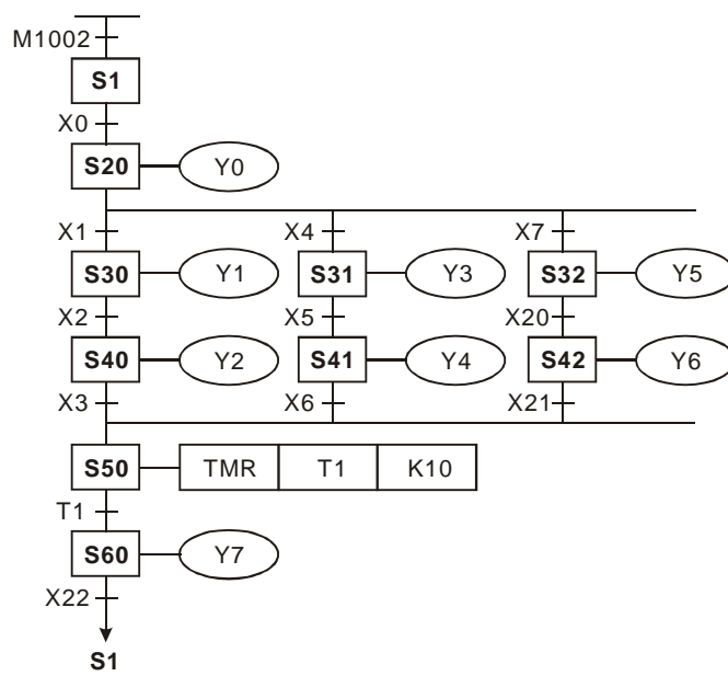
SFC диаграмма:
