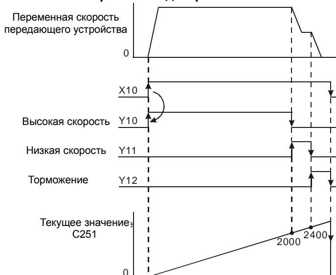
Временная диаграмма
