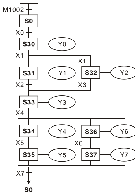
SFC диаграмма:
