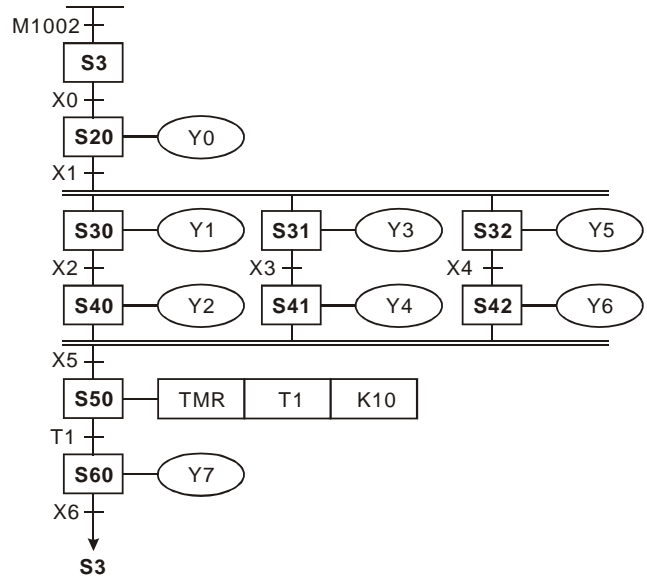
SFC диаграмма:
