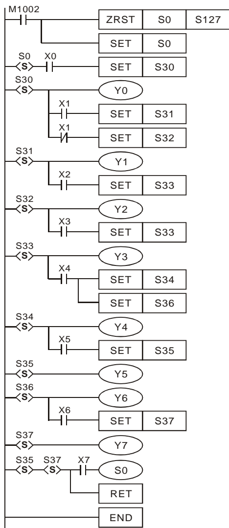
Лестничная диаграмма:
