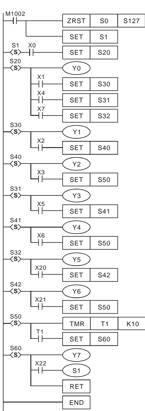
Лестничная диаграмма:
