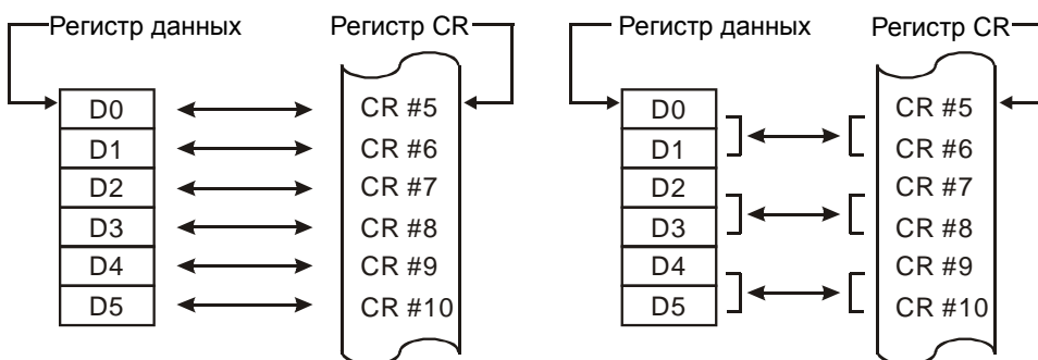
16-битная команда при n=6
