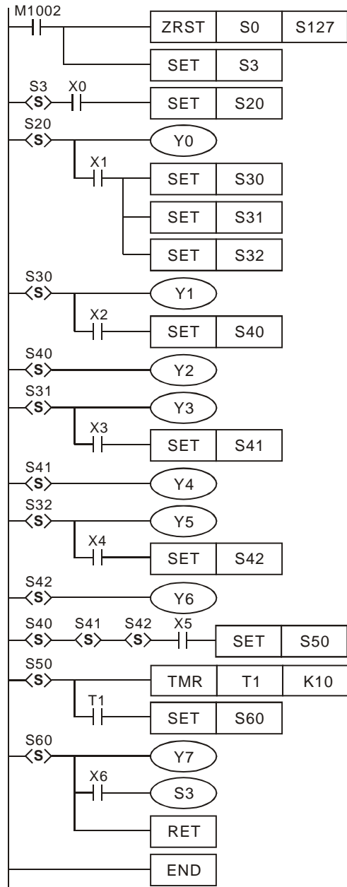
Лестничная диаграмма:
