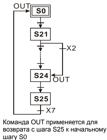
SFC диаграмма:
