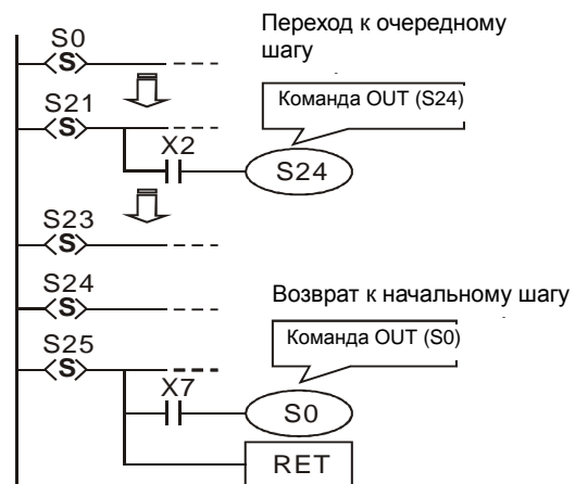
Лестничная диаграмма:
