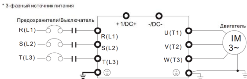
Рисунок 2. Типоразмер D0 и выше
