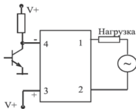
NPN, нормально-разомкнутый
