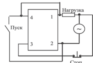
Схема с самоблокировкой (AC-AC)
