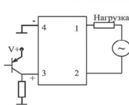
PNP, нормально-разомкнутый
